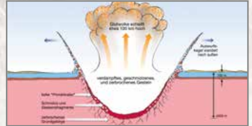
Entstehung des „Primärkraters“ nach etwa 10 Sekunden
