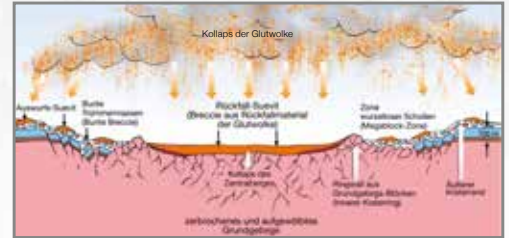
Ende der Kraterbildung und Ablagerung des Suevits nach 10 Minuten
