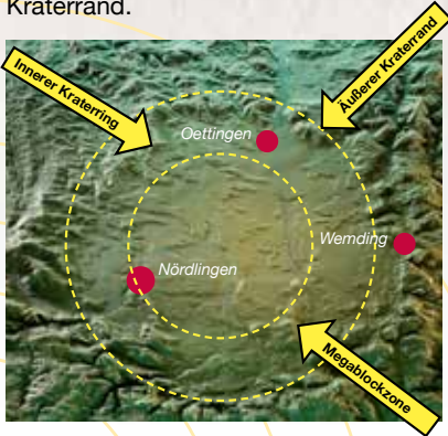
Kollaps des „Primärkraters“ und Ablagerung der Auswurfsmassen nach 1 Minute
