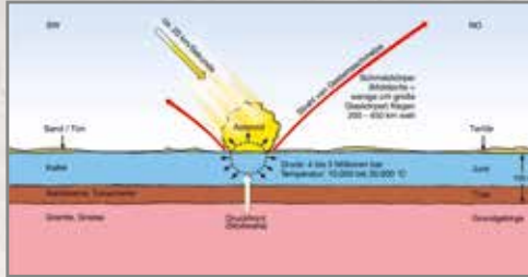
10 Millisekunden nach dem Einschlag
