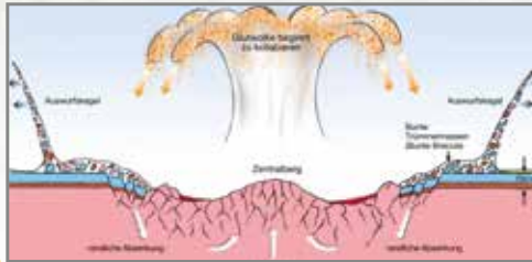
Kollaps des „Primärkraters“ und Ablagerung der Auswurfsmassen nach 1 Minute
